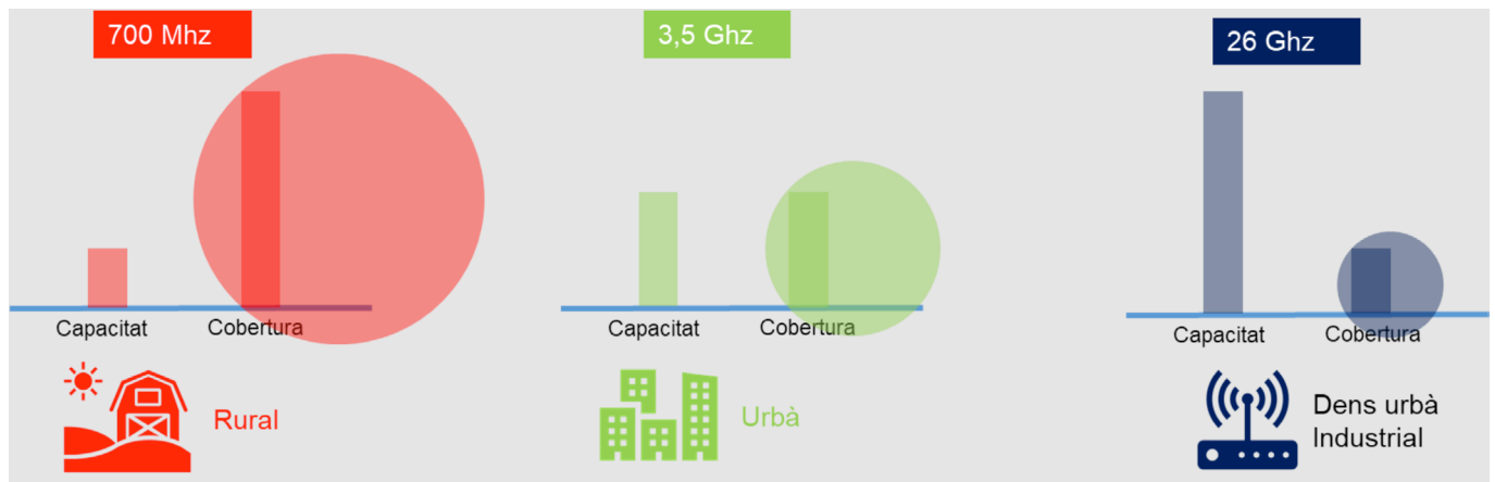
Il·lustració 3: Diferents àmbits necessiten diferents freqüències i proporcionen diferents àrees de cobertura i capacitat
